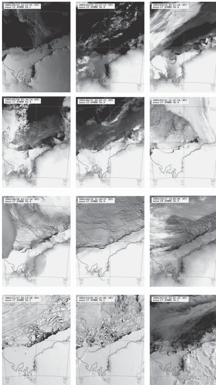
図 1 2005 年 2 月～2006 年 1 月のリュツォ・ホルム湾域の NOAA 衛星画像 Fig. 1. NOAA satellite images of the Lützow-Holm bukta area from February 2005 to January 2006.
