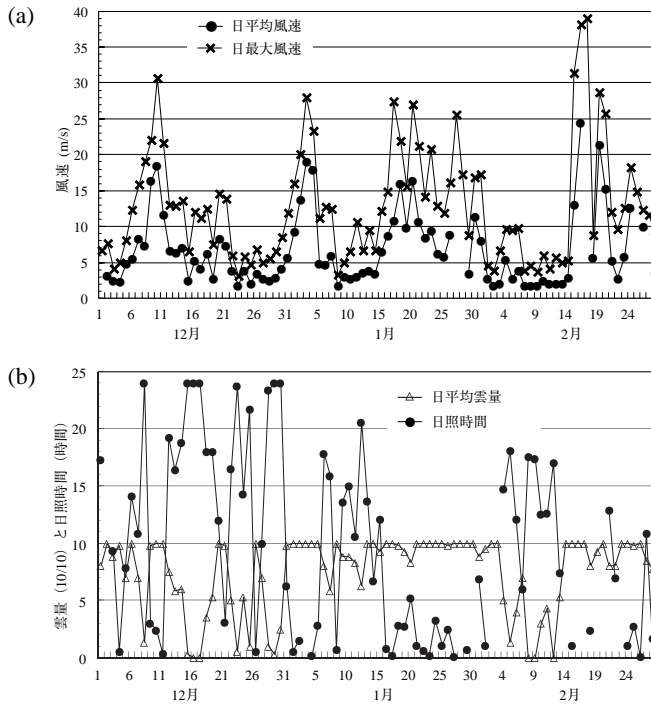
図1 昭和基地における夏の風速 (a) と雲量, 日照時間 (b)。
