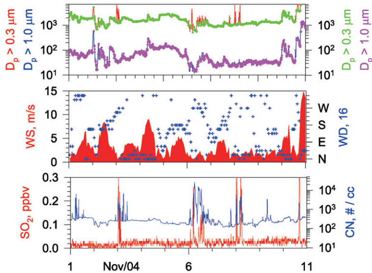
図1 昭和基地における2004年11月1-11日にかけての観測例。上段:スクリーニング前(赤と青)と後(緑と紫)の D_p > 0.3 \mu\text{m} と D_p > 1.0 \mu\text{m} の大気エアロゾル粒子個数濃度,中段:風速(W S:左軸,赤)と風向(W D:右軸,青十字),下段: \text{SO}_2 濃度(左軸,赤)と総エアロゾル粒子数濃度(CN:右軸,青)
