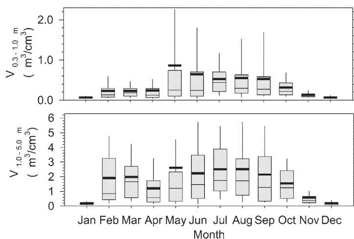
図3 昭和基地における微細粒子 ( D_p 0.3-1.0 \mu\text{m} ) と粗大粒子 ( D_p 1.0-5.0 \mu\text{m} ) の体積濃度の月別変化(2004年2月~2006年1月)。箱ひげ図は、箱の上下が25%と75%のデータ範囲、箱の上下の縦棒の範囲が10%と90%のデータ範囲、箱内の細横線が中央値、太線が平均値をそれぞれ示す。
