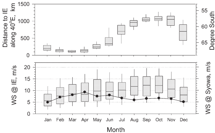
図6 東経40度に沿っての海水縁の位置(上段の箱ひげ図)と海水縁での風速(下段の箱ひげ図)、昭和基地での平均風速(下段の●)。海水縁の位置の統計は、1996-2006年のデータに基づく(牛尾, 2006)。海水縁での風速は、NCEP再解析データセットから925 hPa面についての値。箱ひげ図の表し方はこれまでと同様。
