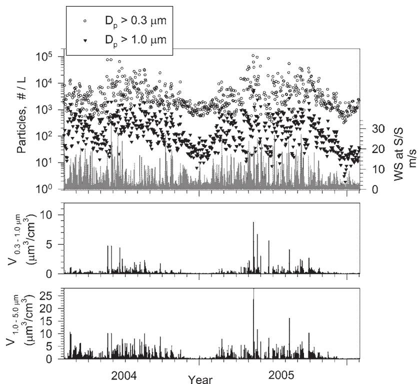
図2 昭和基地における2004年2月～2006年1月までのエアロゾル濃度日平均値。上段: D_p > 0.3 \mu\text{m} (○) と D_p > 1.0 \mu\text{m} (▼) の粒子数濃度(左軸), 風速(右軸, グレー), 中段: V_{0.3-1.0 \mu\text{m}} , 下段: V_{1.0-5.0 \mu\text{m}} .
