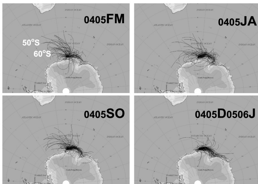
図5 昭和基地付近から2日間遡った後方流跡線。2004年2月~2006年1月にかけての(左上):2-3月,(右上):7-8月,(左下):9-10月,(右下):12-1月について解析した結果。
