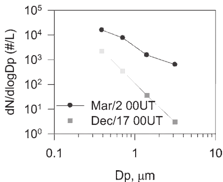
図7 2004年3月2日と12月17日に昭和基地で得られた個数粒径分布 Fig. 7. Number size distributions on March 2 and December 17, 2004 at Syowa Station.
