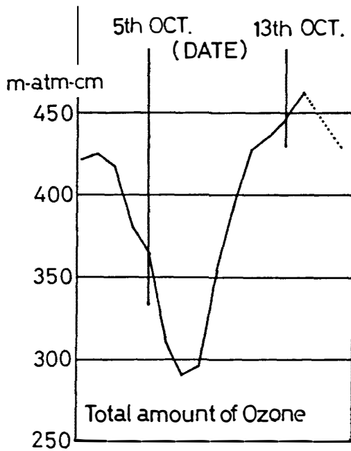
図 10 オゾン全量の変化 (突然昇温期, 1979年10月) Fig. 10. Total amount of ozone in the sudden warming period (October 1979).
