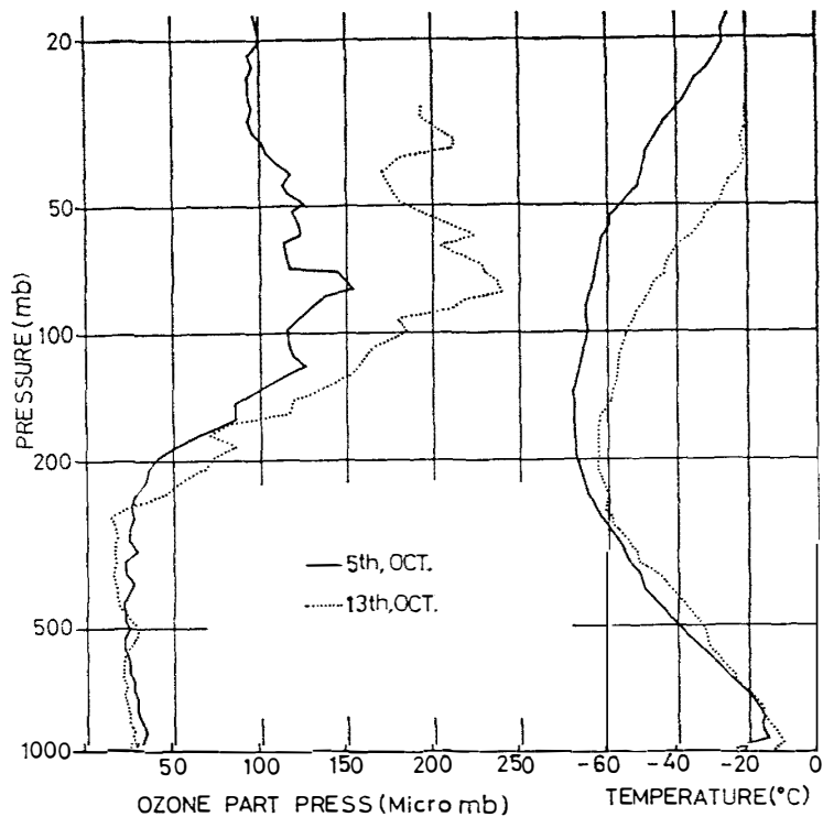
図 9 突然昇温前後のオゾンゾンデ観測結果 Fig. 9. Examples of ozone sonde observation in the sudden warming period.
