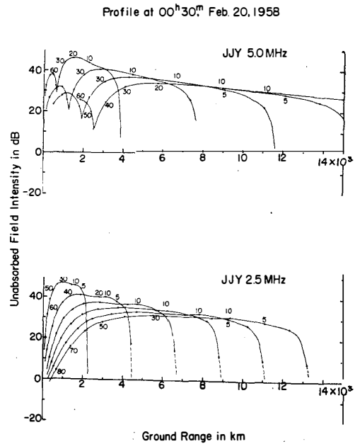
図 4 (b) プロファイル M に対して, JJY 5 と 2.5 MHz の諸量を与えて計算した無減衰電界強度(図中の数字は発射角度)
