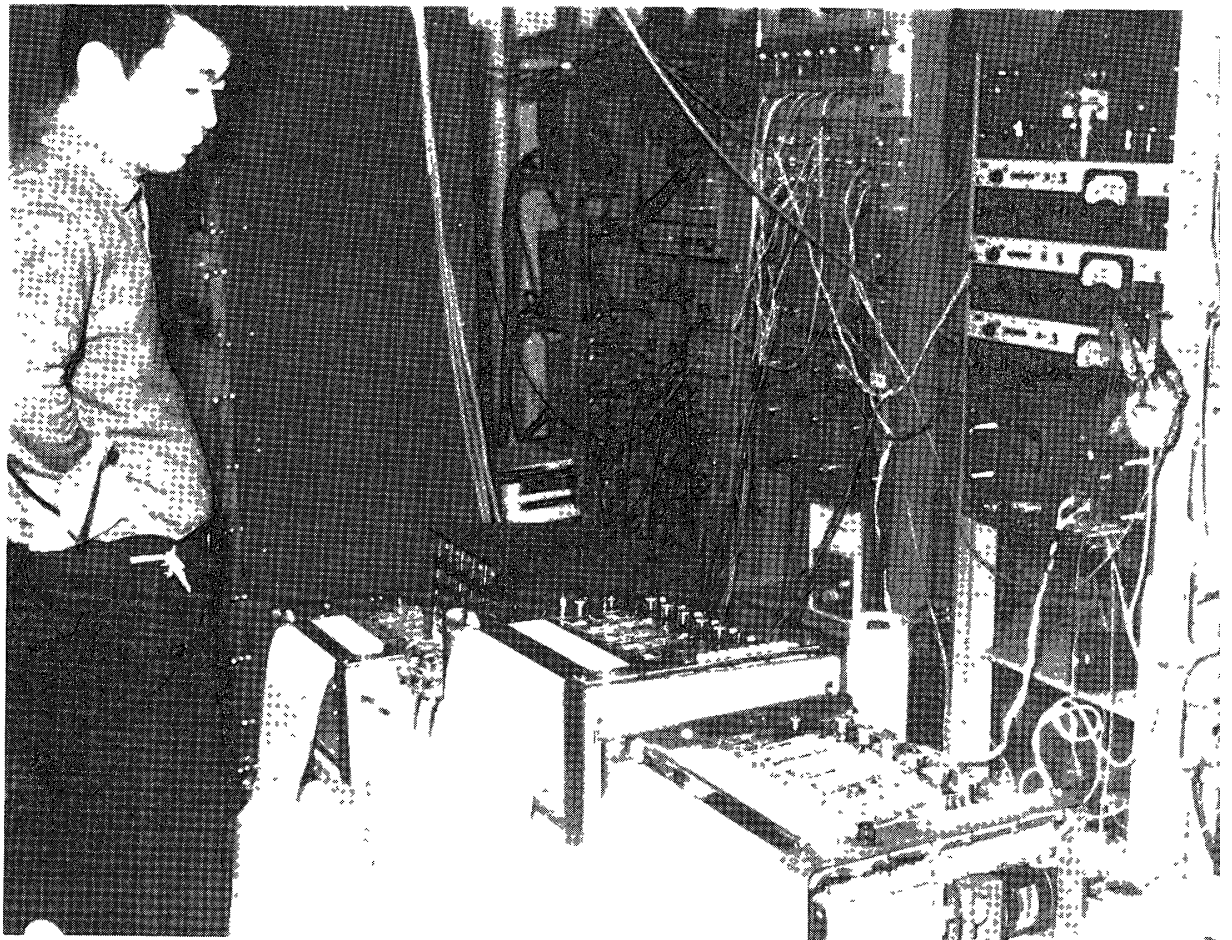
図 2 新視測棟内のオーロラ・地磁気・電波観測装置
