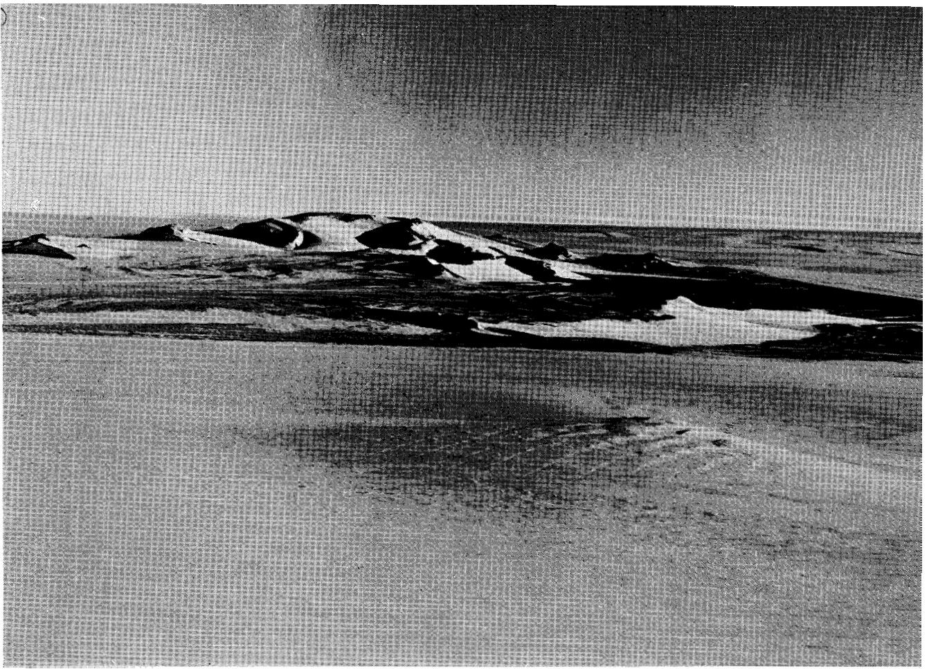
Photo. 13. A photograph showing the northern side of A group. 写真 13. B 頂上から A の北面を望む.
