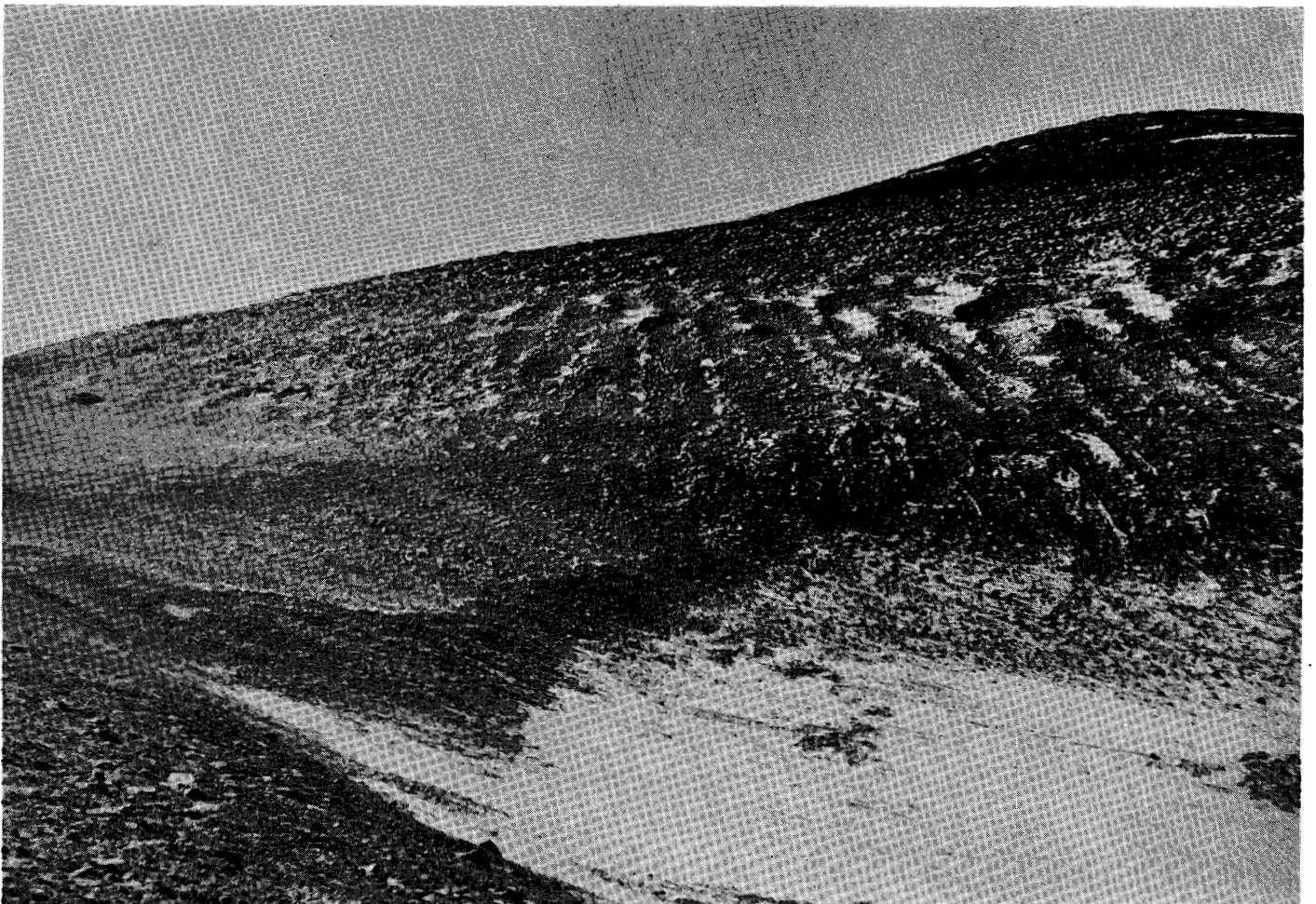
Photo. 14. Stone stripes formed on the broad ridge of B group. 写真 14. B の山稜の moraine に形成された stone stripe.
