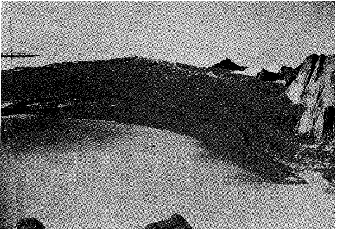
写真 7. 福島岳西側の大圏谷氷河を、圏谷壁の上から見おろす.
