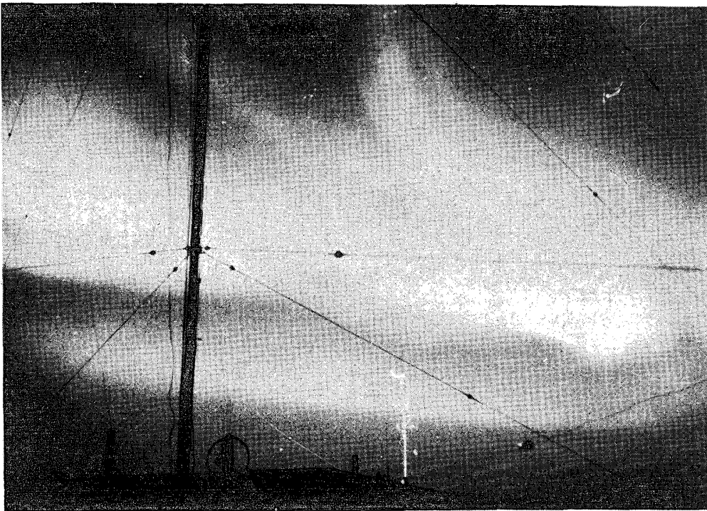
Active Aurora. 01 : 00, Aug. 2, 1959.
