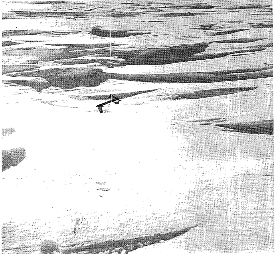
写真 16-3 浸蝕が進んで、この場合深さ約 40 cm あつた積雪層の底面が露われるほどにまで成長した。サストルギの高さ 25~40 cm, 表面のザラザラした面 (例えばピッケルの置いてあるところ) は一年氷の最上面を示す。
