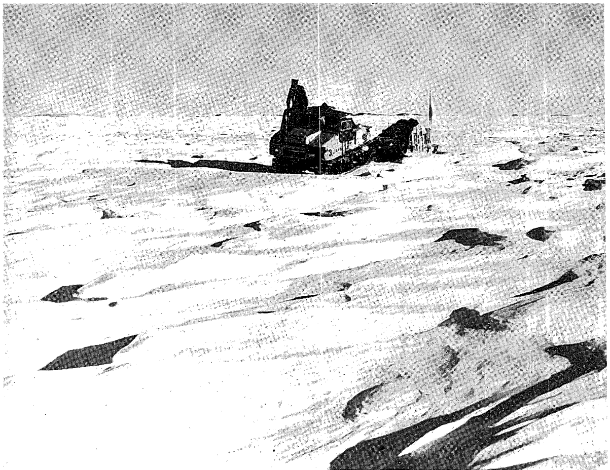
写真 16-4 高さ 30~70 cm のサストルギの一面に発達した海水原。
