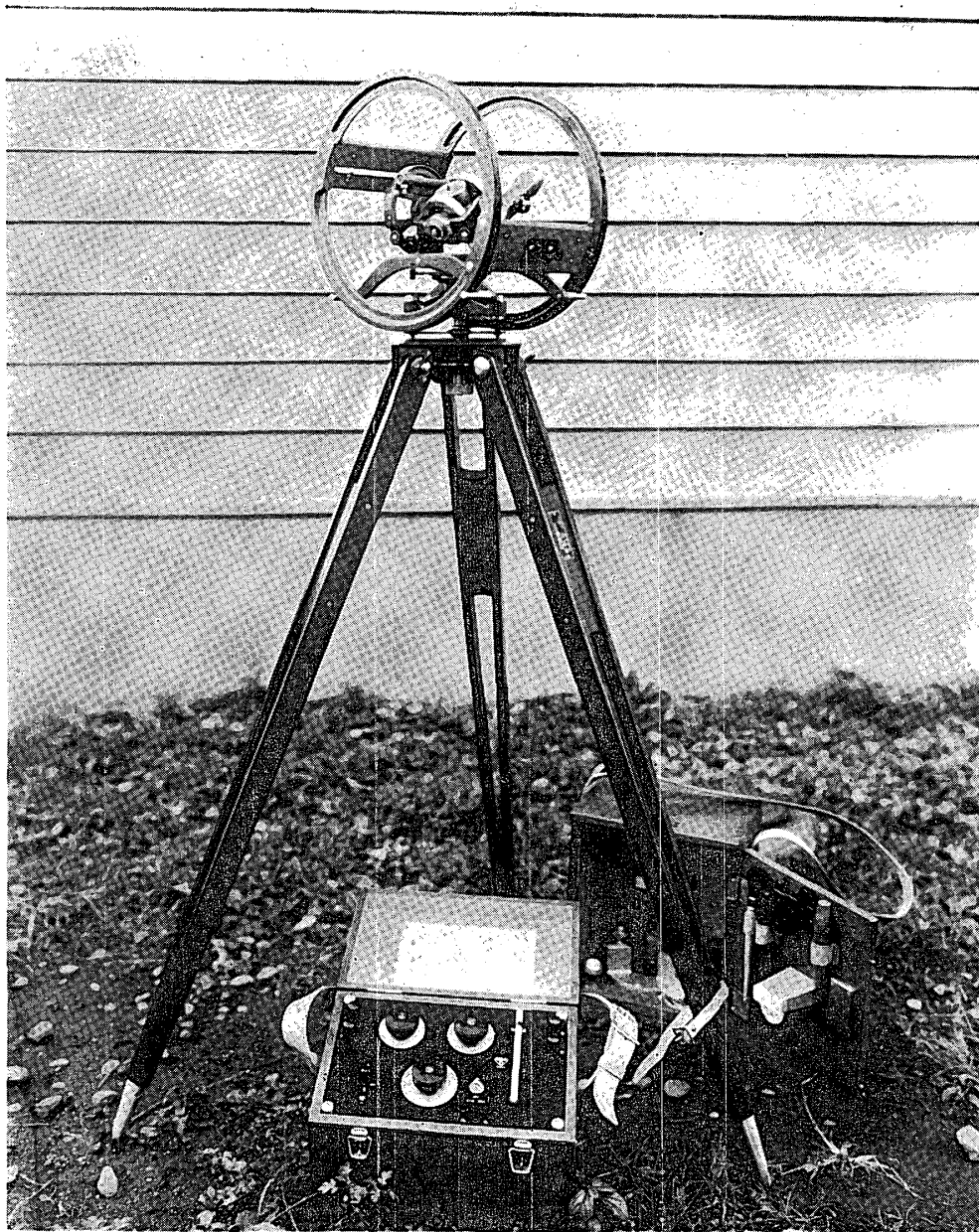
写真 1 地震研究所型磁力計
