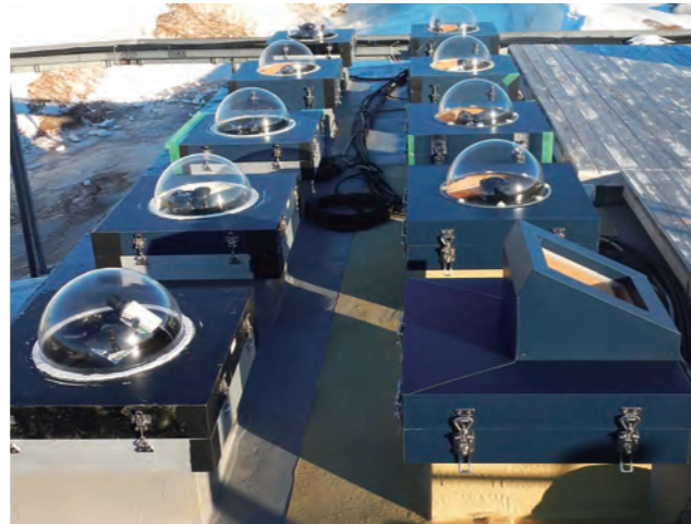
昭和基地のオーロラ光学観測機器
