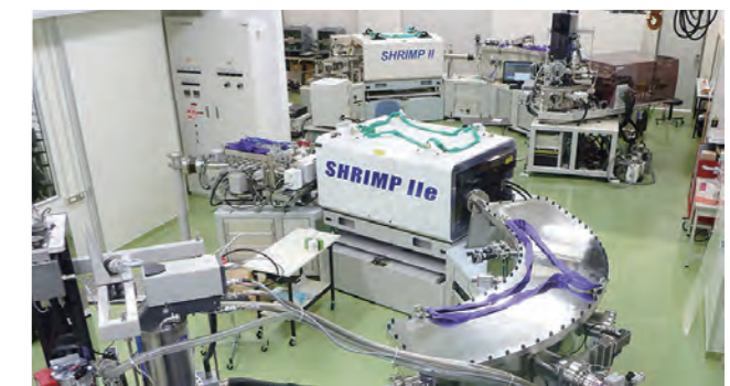
鉱物の年代測定を行う二次イオン質量分析計 (SHRIMP)
