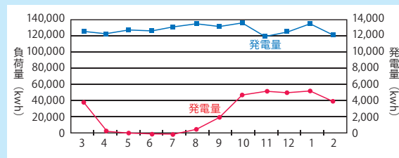
昭和基地における使用電力量と太陽光発電量
