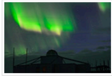
昭和基地のオーロラ (photo : JARE54)
