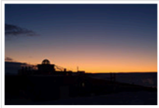
昭和基地の黎明 (photo : JARE53)
