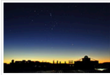
昭和基地とオリオン座 (photo : JARE50)
