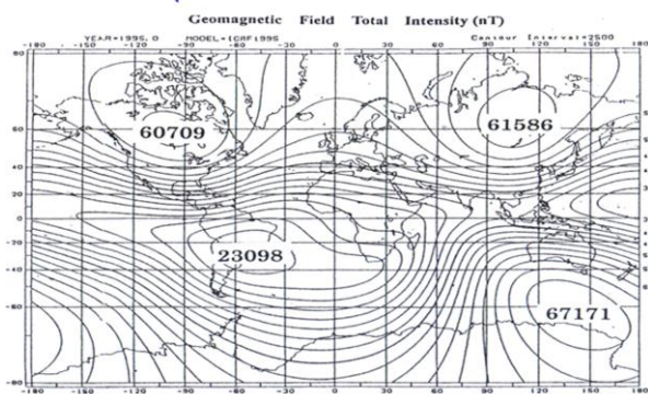
1995 IGRF Model
